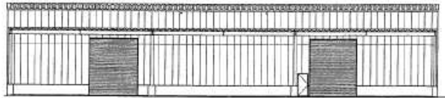
東立面図
